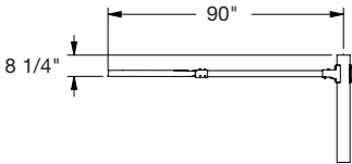
16-A, 20-A, 25-A, 30-A CLB-SS-53 Weight: 35.7 lbs
